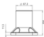
vooraanzicht
