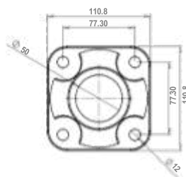
bovenaanzicht
