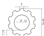
vooraanzicht
