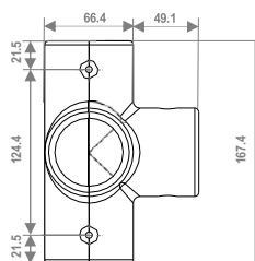
vooraanzicht
