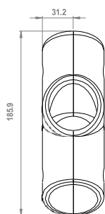
bovenaanzicht
