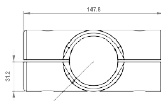
bovenaanzicht
