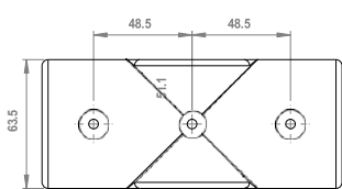
vooraanzicht
