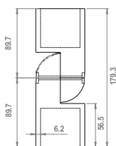
vooraanzicht
