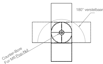
zij aanzicht
