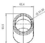
vooraanzicht
