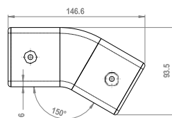
zij aanzicht
