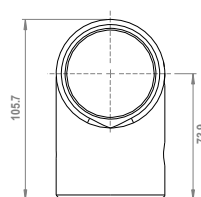
zij aanzicht
