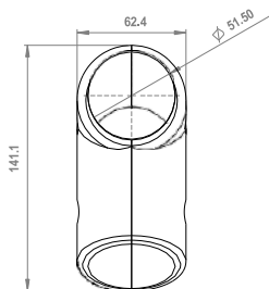
vooraanzicht
